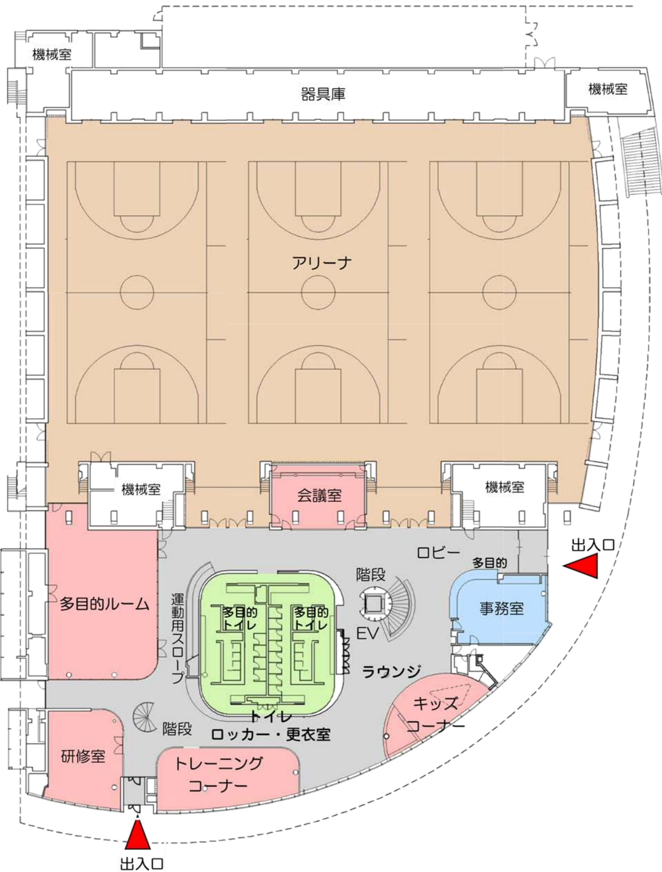
1階平面図
